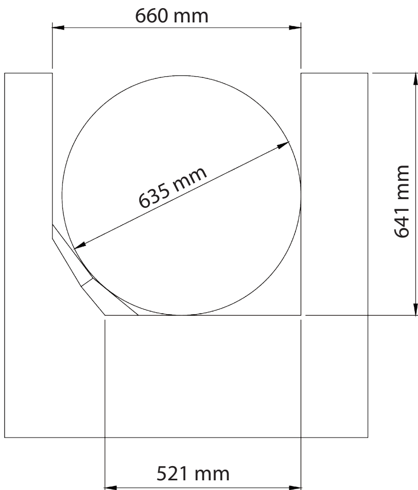
Calha do Picador de 96"
